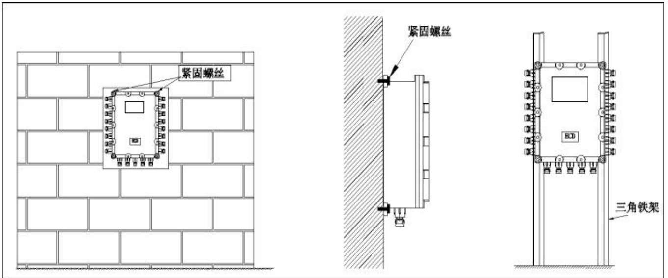
图 2、报警控制器安装图
